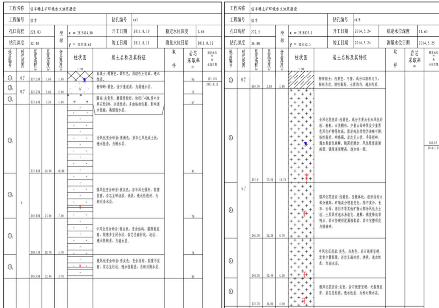
图 3.2.2-1 赣县韩坊、信丰赤岗、窑下稀土矿环境水文地质勘查钻孔柱状图
