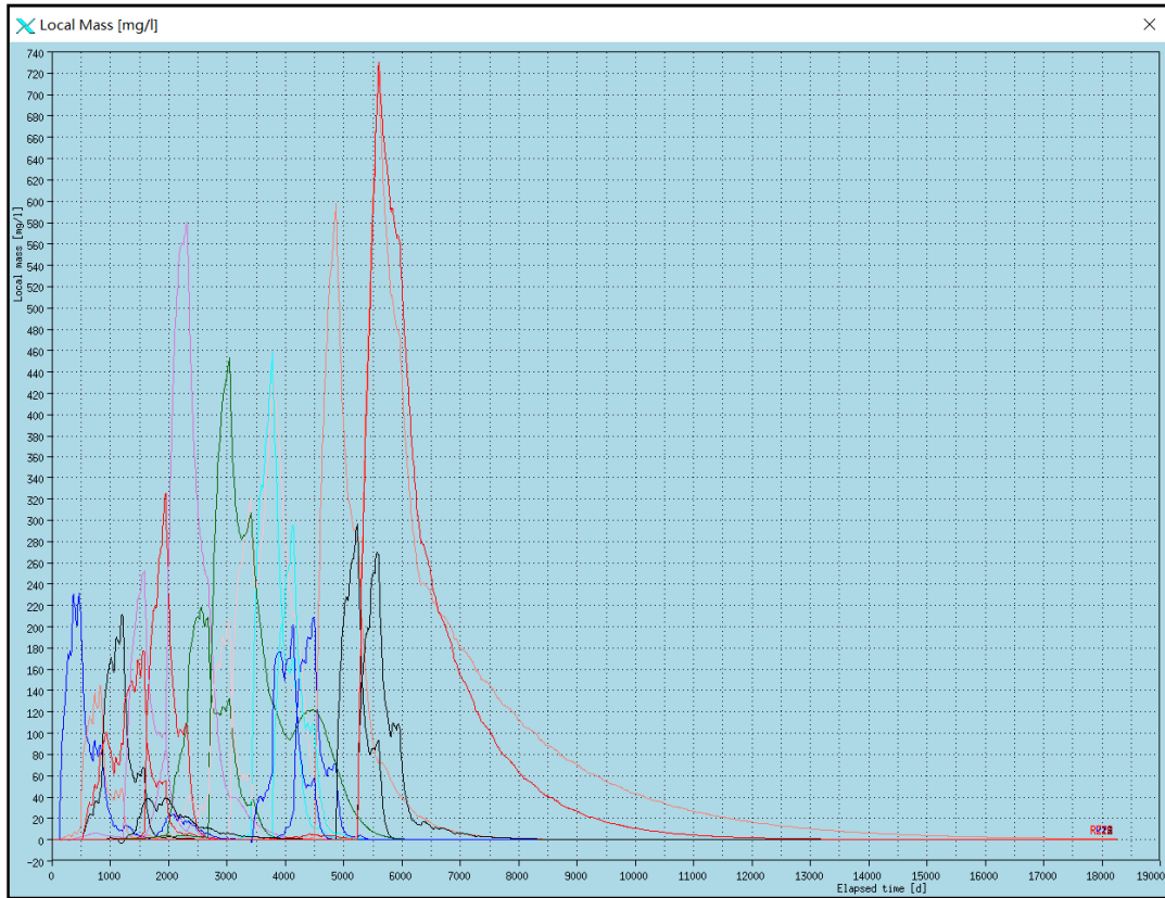
图 5.2.4-2 大埠矿区矿块开采镁离子浓度随时间变化曲线图
