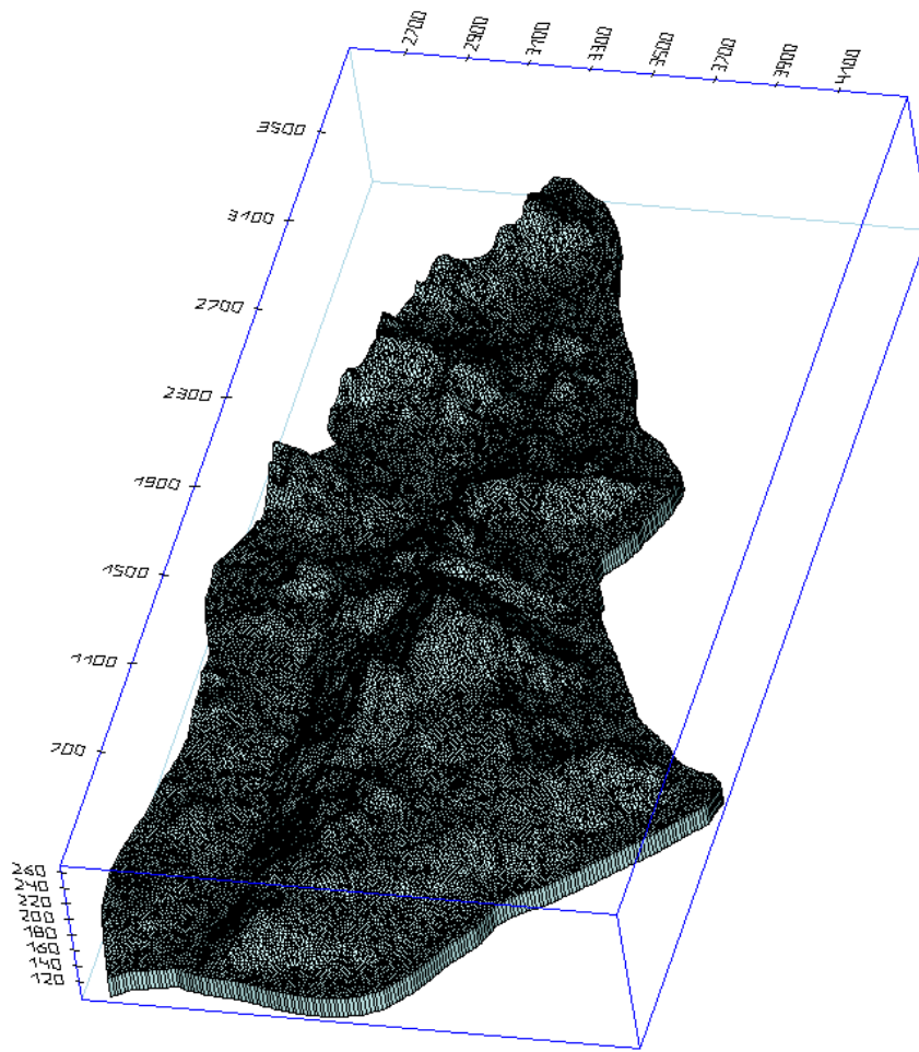
图 5.2.2-2 地下水渗流模型的网格剖分立体图
