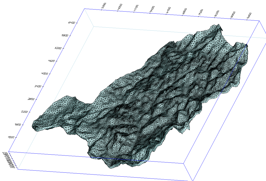
图 5.3.2-2 地下水渗流模型的网格剖分立体图
