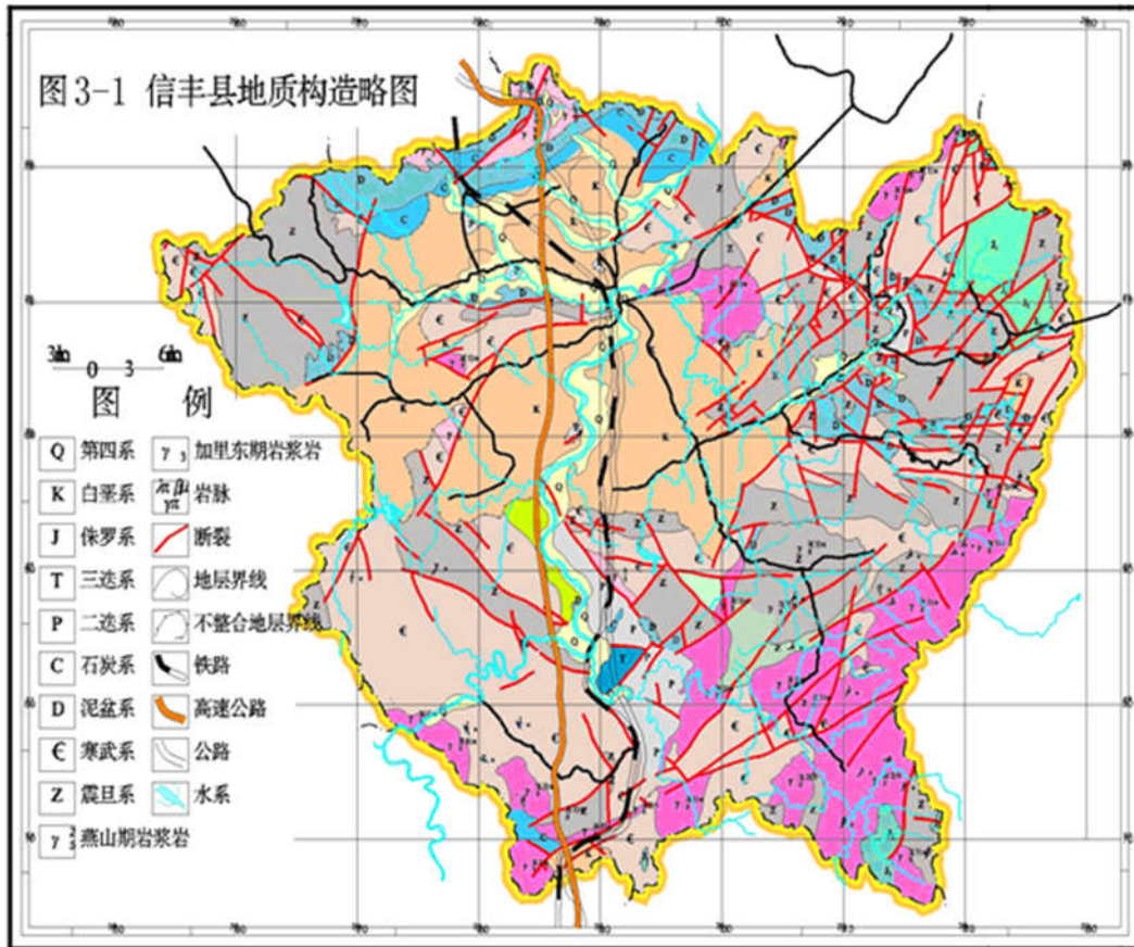
图 2.4.1-1 地质构造
