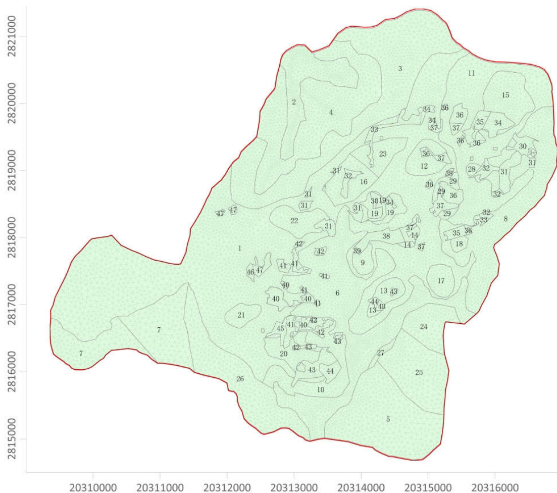
图 5.3.2-3 韩坊坑模拟区降雨入渗系数分区
