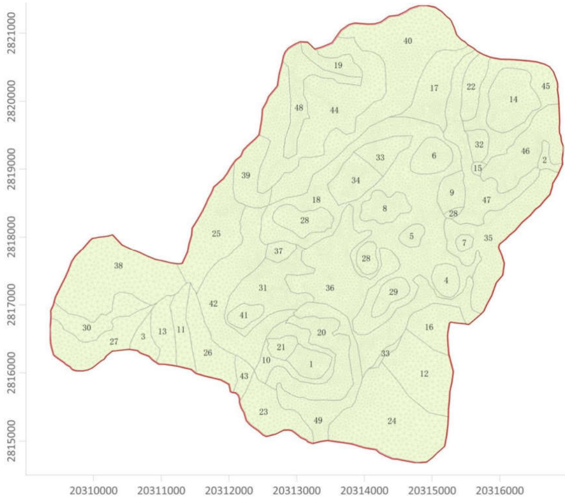
图 5.3.2-4 韩坊模拟区含水层渗透系数分区
