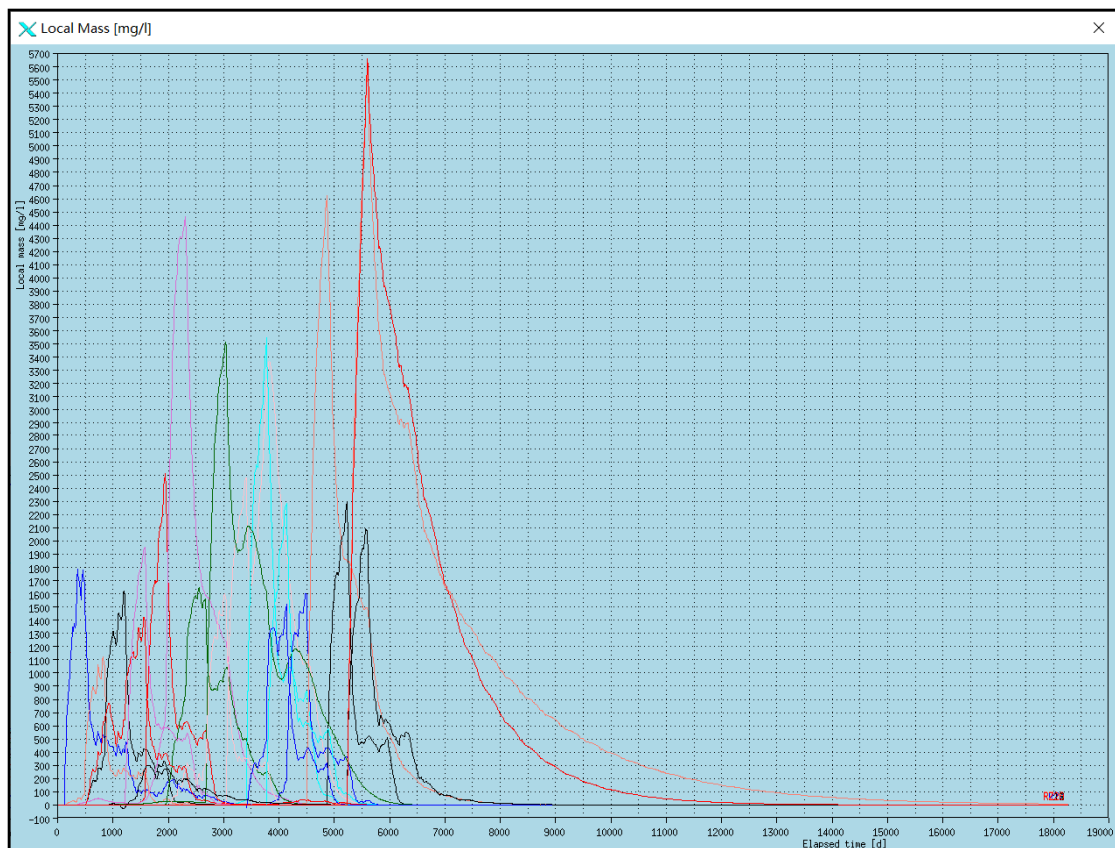
图 5.2.4-4 大埠矿区矿块开采硫酸根离子浓度随时间变化曲线
