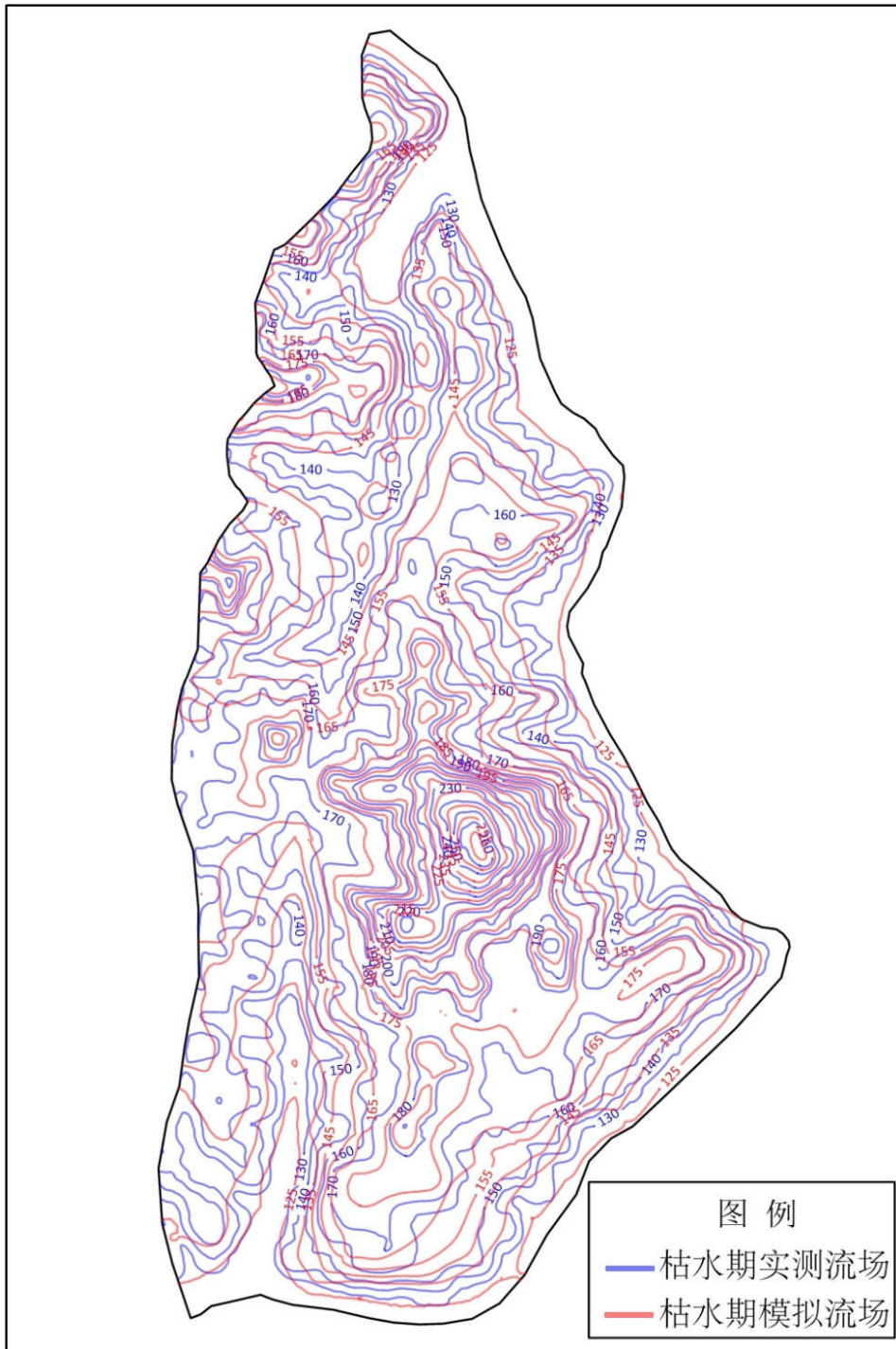
图 5.2.2-6 模拟区枯水期实测等水位线与计算等水位线对比图 (2021.11)
