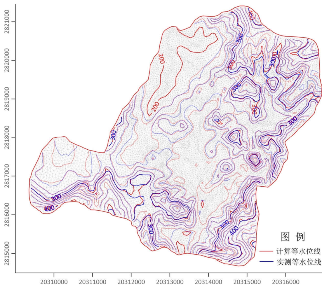
图 5.3.2-6 模拟区枯水期实测等水位线与计算等水位线对比图 (2021.11)
